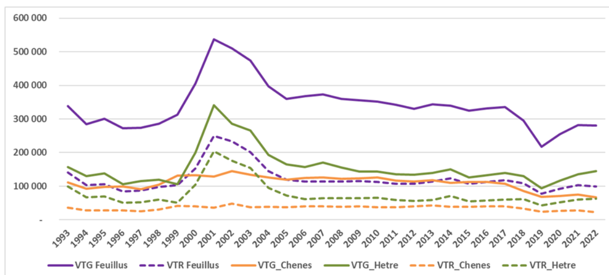
Figure 4.17. Évolution du Volume Total Global (VTG) et du Volume Total des Reliquats (VTR) pour les tous les feuillus et les deux essences dominantes (chênes et hêtres).
