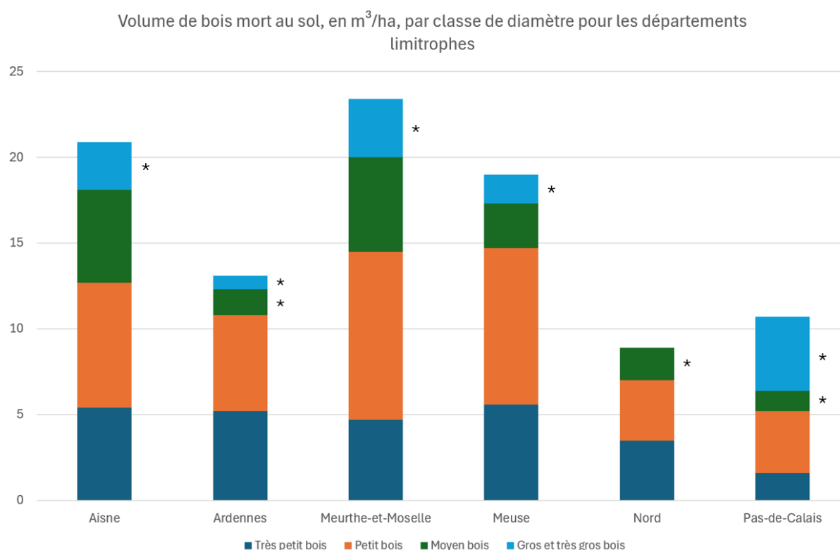
Figure 4.7. Volume de bois mort au sol, en m 3 /ha, en fonction des classes de diamètre dans les départements limitrophes à la Wallonie pour la période allant de 2014 à 2023 15 . Les classes de diamètre correspondent à : très petit bois entre 2,5 et 7,5 cm, les petits bois entre 7,5 et 22,5 cm, les moyens bois entre 22,5 et 37,5 cm et les gros et très gros bois avec un diamètre supérieur à 37,5 cm. Les * signifient que ces valeurs possèdent un intervalle de confiance important.
