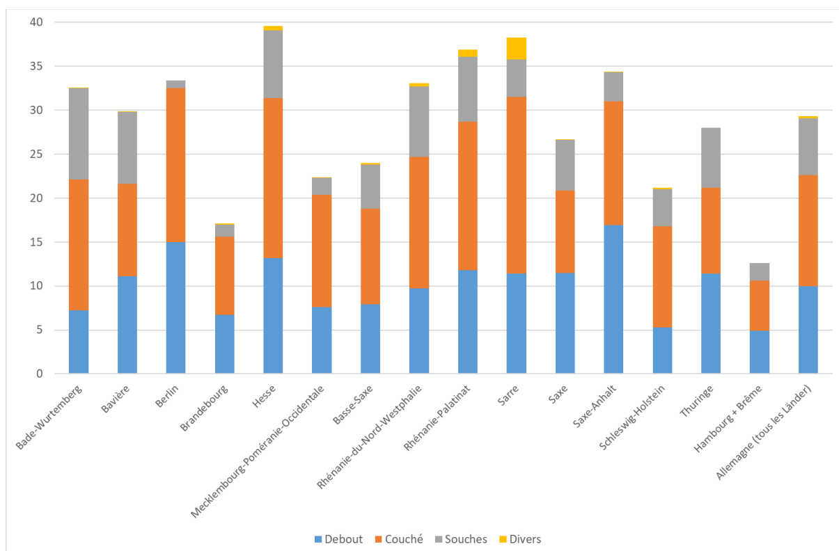
Figure 4.2. Répartition des volumes moyens de bois mort en différentes catégories, debout, couché, souches et restes divers, dans les forêts allemandes en 2022.
