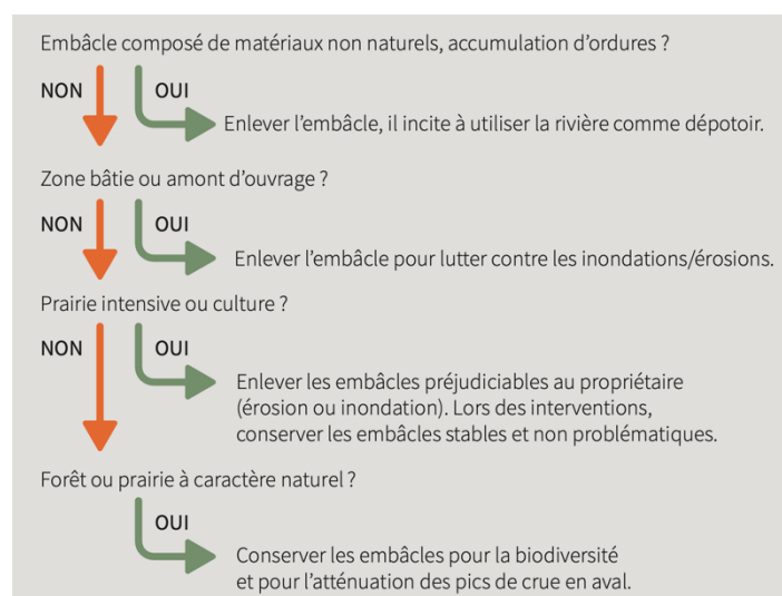
Figure 3.10. Clé décisionnelle pour l'enlèvement ou non du bois en décomposition dans l'eau. D'après (Huylenbroeck et al., 2019).
