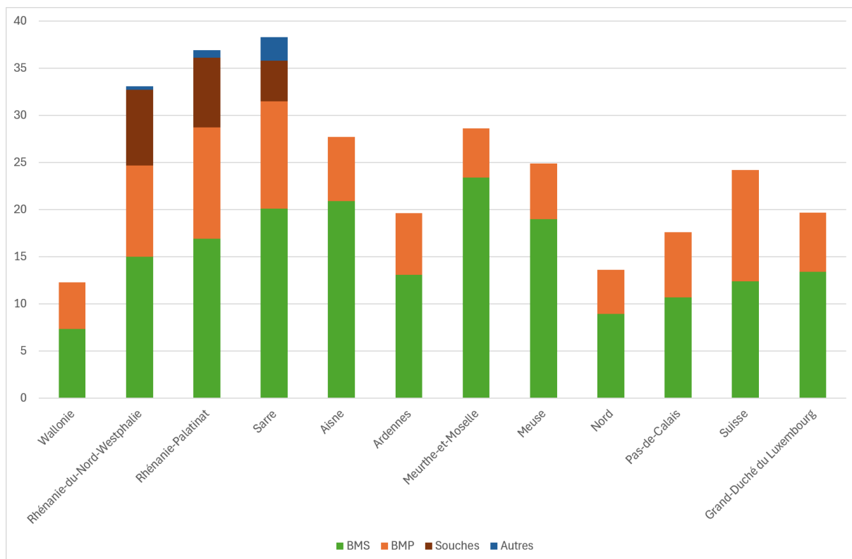
Figure 4.15. Volume, en m 3 /ha, de bois mort, sur pied, au sol, dans les souches et divers, pour la Wallonie et les différents pays et régions voisins. Pour l'Allemagne, les chiffres correspondent aux 3 régions voisines : Rhénanie-du-Nord-Westphalie, Rhénanie-Palatinat et Sarre. Pour la France, les chiffres correspondent aux 5 départements voisins : Aisne, Ardennes, Meurthe-et-Moselle, Meuse, Nord et Pas-de-Calais.
