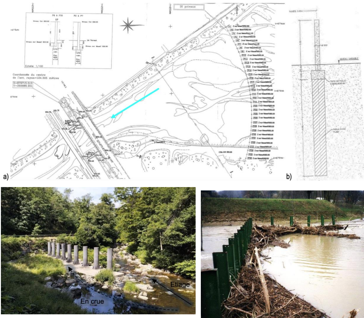
Figure 3.8. Différents exemples de pièges à flottants mis en place en France. D'après (Benaksas & Piton, 2023).
