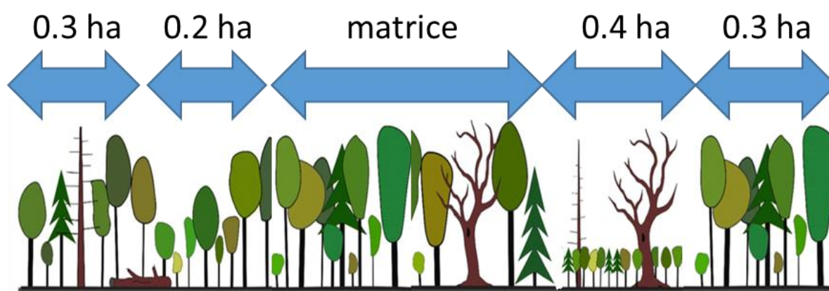
Figure 7.8. Essai de représentation de la logique des mailles de 0.3 ha qui sont générées (mais pas aussi densément !) dans les forêts domaniales de Sarre pour mimer la structure des forêts naturelles.
