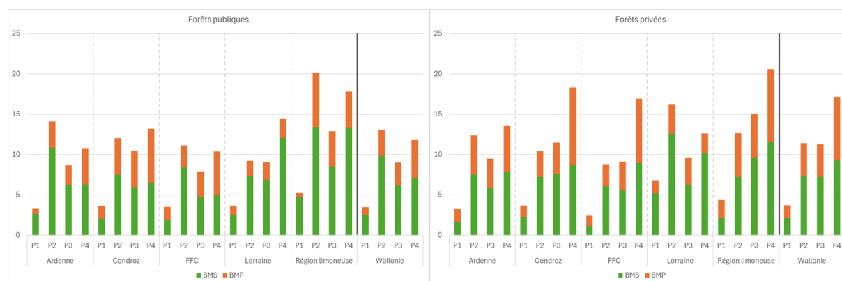
Figure 4.13. Volume, en m 3 /ha, de bois mort, sur pied et au sol, pour les différentes régions biogéographiques de Wallonie. A gauche, les forêts publiques et à droite, les forêts privées. Ces volumes sont répartis en fonction de la période de récolte des données (P1 = 1994-2000, P2 = 2001-2008, P3 = 2008-2015, P4 = 2015-2023).
