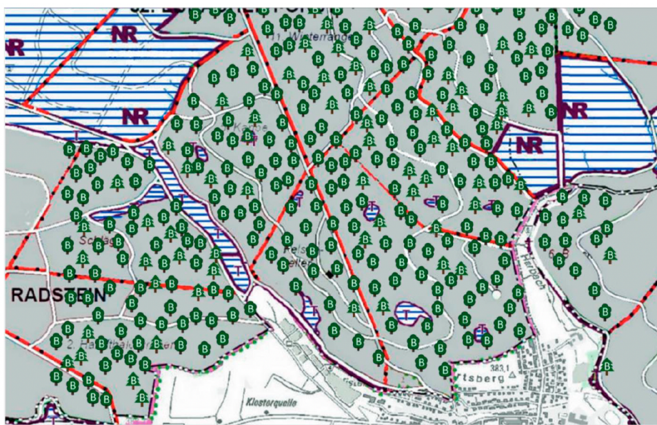
Figure 7.15. Cartographie d'une partie de la forêt montrant la structuration spatiale du réseau des zones en libre évolution avec les réserves intégrales forestières (NR), les îlots de sénescence (T) et du réseau des Arbres-Habitats (B) jouant le rôle de « pas japonais ».
