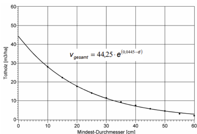
Figure 4.4. Relation entre le diamètre minimum d'inventaires et les volumes de bois mort par hectare.
