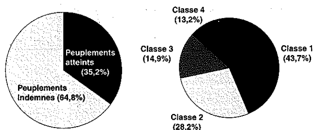
Figure 1. - Ventilation des pessières wallonnes selon l'intensité des dégâts de gibier observée.
