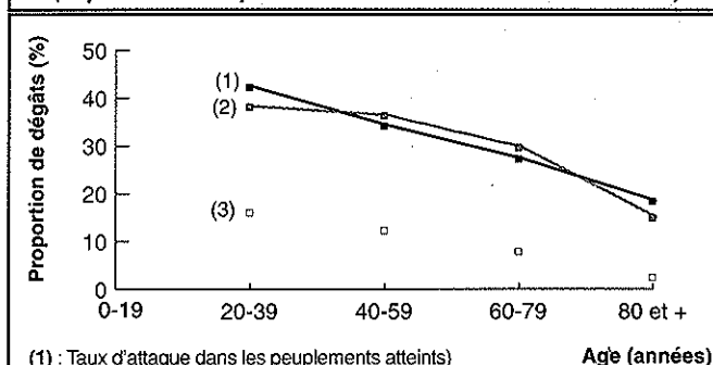
Figure 2. - Evolution des dégâts de gibier selon l'âge (exprimée en fréquences relatives des surfaces atteintes).
