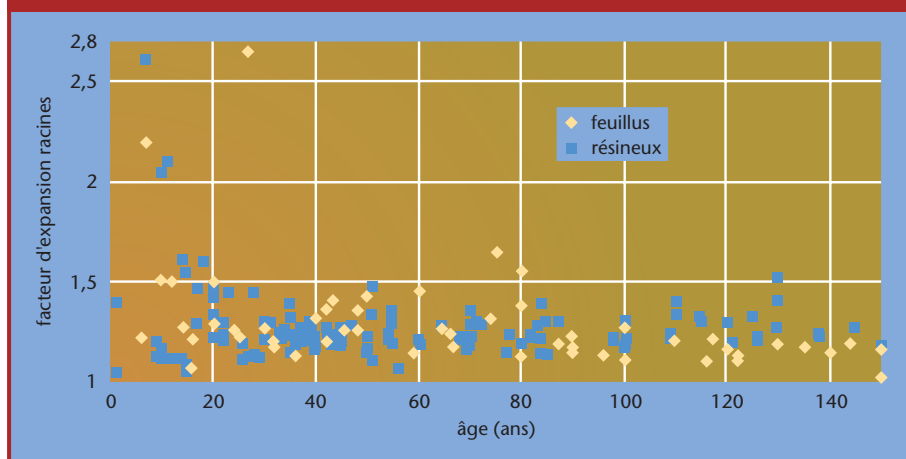
Figure 2 – Variabilité du facteur d'expansion racines (rapport de la masse totale ligneuse du peuplement à sa masse ligneuse aérienne) d'après l'analyse bibliographique de 240 peuplements des zones tempérées boréales et méditerranéennes 3-5
