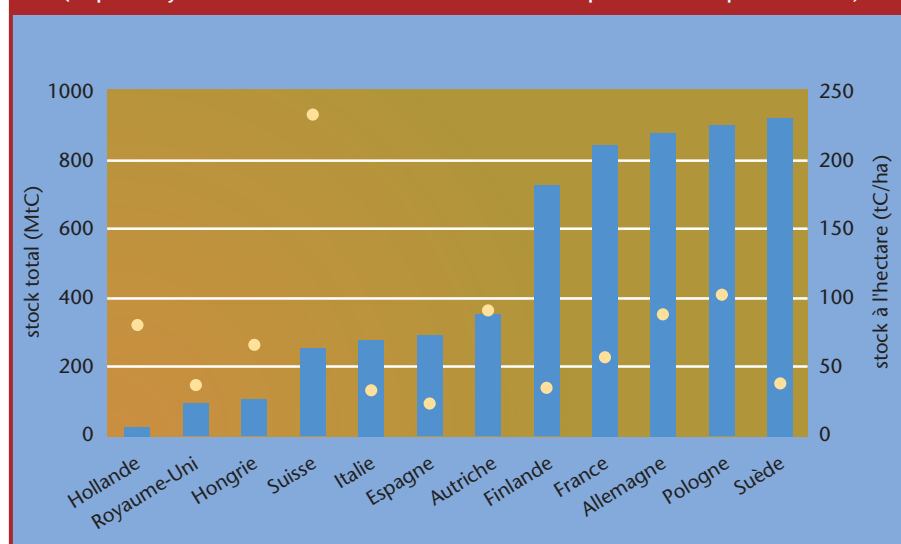
Figure 4 – Stocks totaux (barres) et à l'hectare (points) de carbone dans la biomasse forestière de quelques pays européens (d'après la synthèse de NABUURS et al. 11 et les données de la présente étude pour la France)
