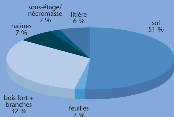
Figure 5 – Répartition du carbone des forêts françaises dans les différents compartiments de l'écosystème (total de 137 tC/ha)
