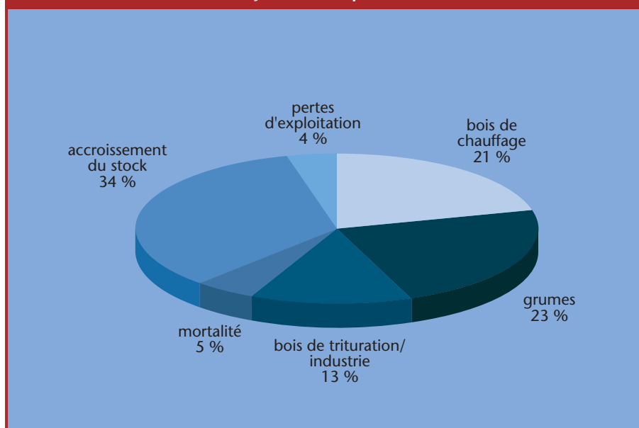
Figure 7 – Devenir de la production moyenne en volume des forêts françaises sur la période 1979 – 1991
