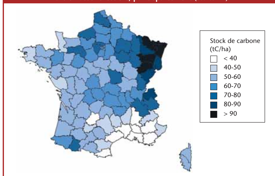
Figure 3 – Stock moyen de carbone par unité de surface dans la biomasse forestière, par département (Source IFN)
