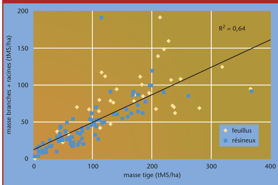
Figure 1 – Relation entre la biomasse des branches et racines et celle de la tige (bois fort sur écorce) dans 119 peuplements des forêts tempérées, boréales et méditerranéennes d'Europe 3
