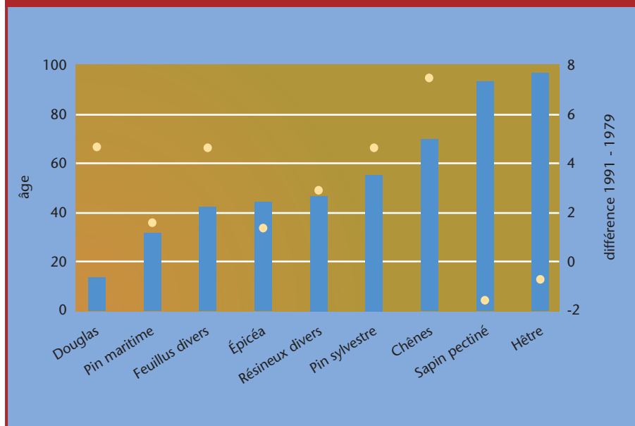
Figure 6 – Âge moyen pondéré par les surfaces des futaies françaises (barres) et variation de cet âge entre 1979 et 1991 (points)
