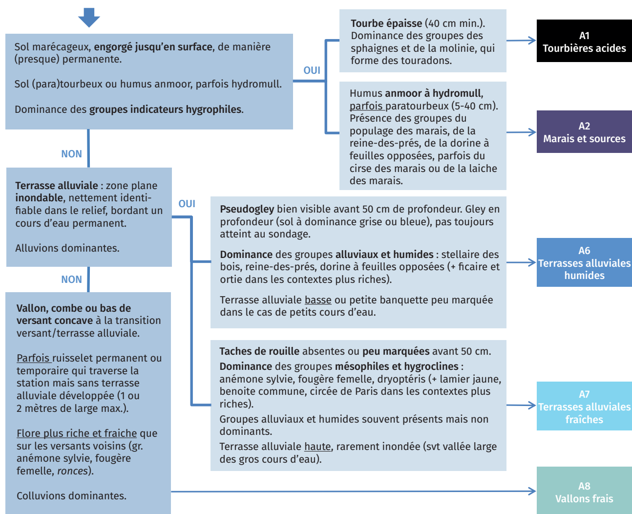
Figure 2. Extrait de la clé d'identification des types de station d'Ardenne, sous-clé des situations alluviales.
