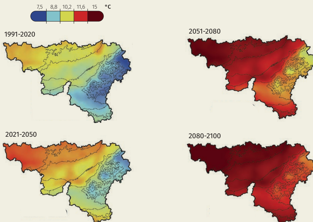
Figure 3. Aperçu de l'évolution des températures moyennes simulées sur les prochaines décennies par le Modèle Atmosphérique Régional (forcé par MPI, CMC et IPL) adapté au scénario SSP5-8.5 du GIEC 4 . Ce scénario considère que les émissions de gaz à effet de serre ne diminueront pas à l'échelle mondiale. Si les gouvernements respectent leurs engagements de réduction des émissions, l'évolution des températures représentée ici sera moins marquée.
