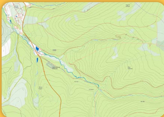
Relief des environs du fourneau Saint-Michel (carte IGN).
