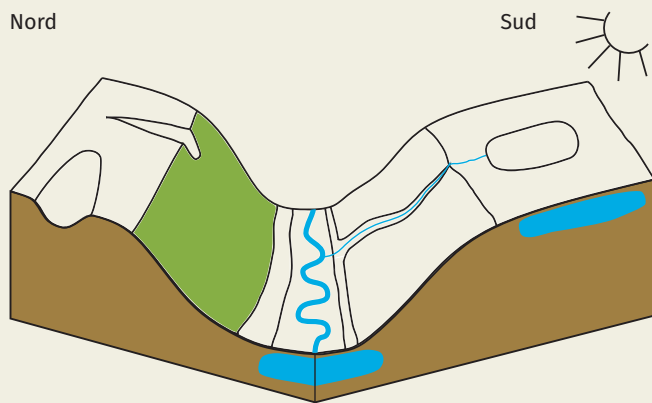
Figure 4. Schéma topographique, illustrant où se rencontre le type de station dans le paysage. Exemple des versants chauds au sol superficiel (type de station A10, avec « A » pour Ardenne).
