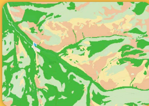
Carte de vulnérabilité des types de station face aux changements climatiques, dérivée de la carte des types de station.
