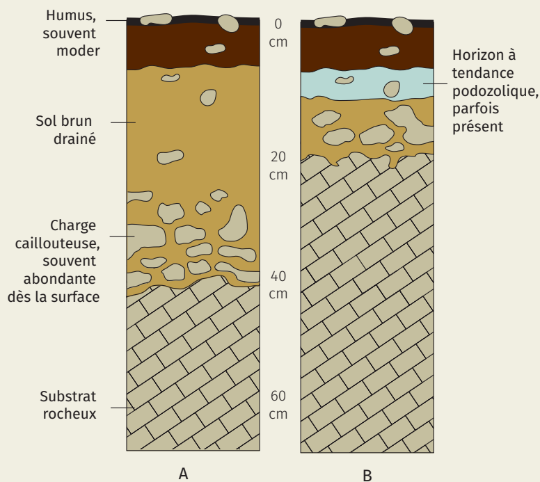
Figure 5. Schéma des profils de sol typiques rencontrés sur le type de station concerné, exemple du type de station des versants chauds au sol superficiel (type de station A10, avec « A » pour Ardenne).
