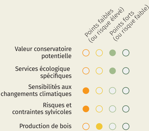
Figure 7. Pictogramme de synthèse des potentialités du type de station, exemple des versants chauds au sol superficiel (type de station A10, avec « A » pour Ardenne).
